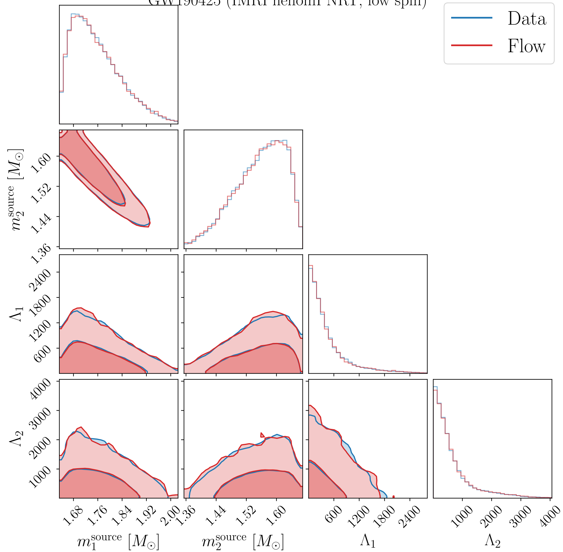
GW190425 (IMRPhenomPNRT, low spin)
